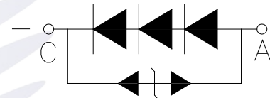
Fig.1-4 Polarity 极性
