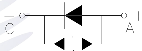
Fig.1-4 Polarity 极性
