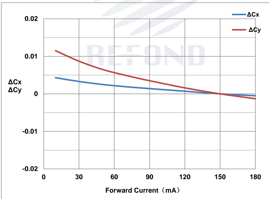
Fig. 1-14 Chromaticity Coordinate Shift Vs Forward Current 色坐标偏移与正向电流特性曲线
