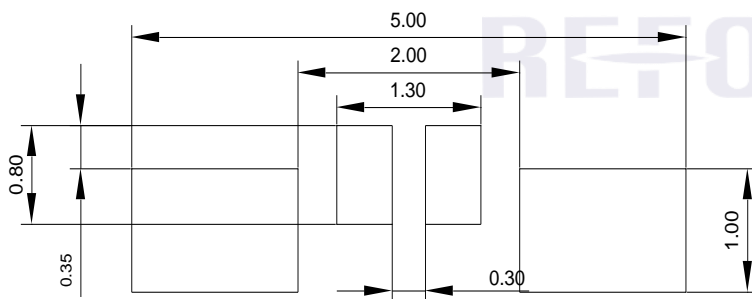
Fig.1-3 Bottom view 背面视图
