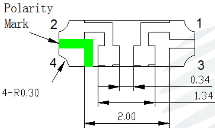
Fig.1-3 Bottom view 背面视图
