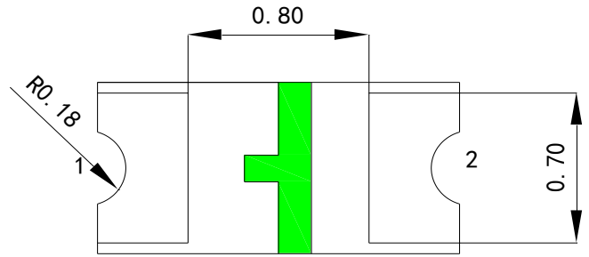
Fig.1-2 Side view 背面视图
