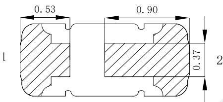
Fig.1-3 Bottom view 背面视图
