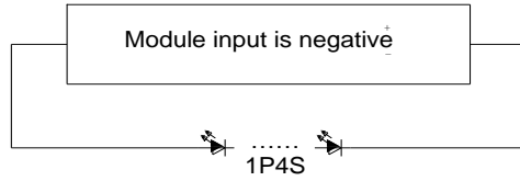
Fig.2-2ED Moduleconnection 模组电性图
