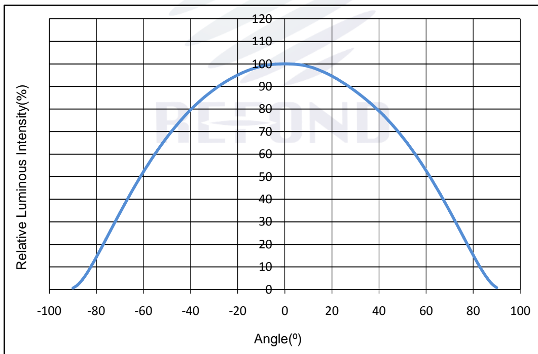
Fig 1-14 Radiation diagram 辐射特性曲线
