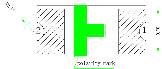
背面视图
